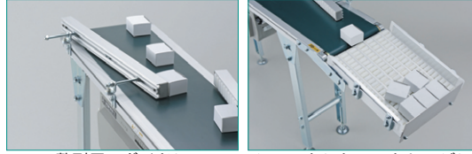
整列用のガイドに
