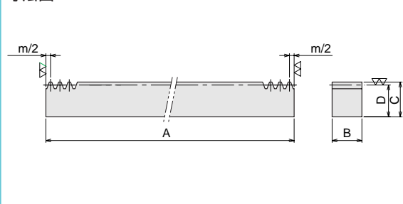
寸法図
